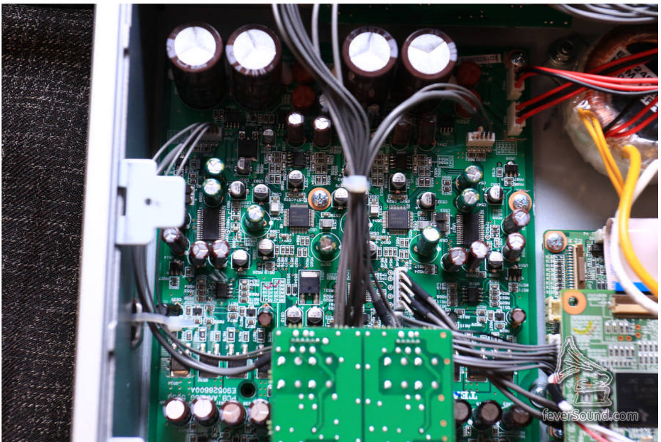
解碼及 Analog Stage，左右聲道獨立分開，AKM 解碼也用上兩粒
